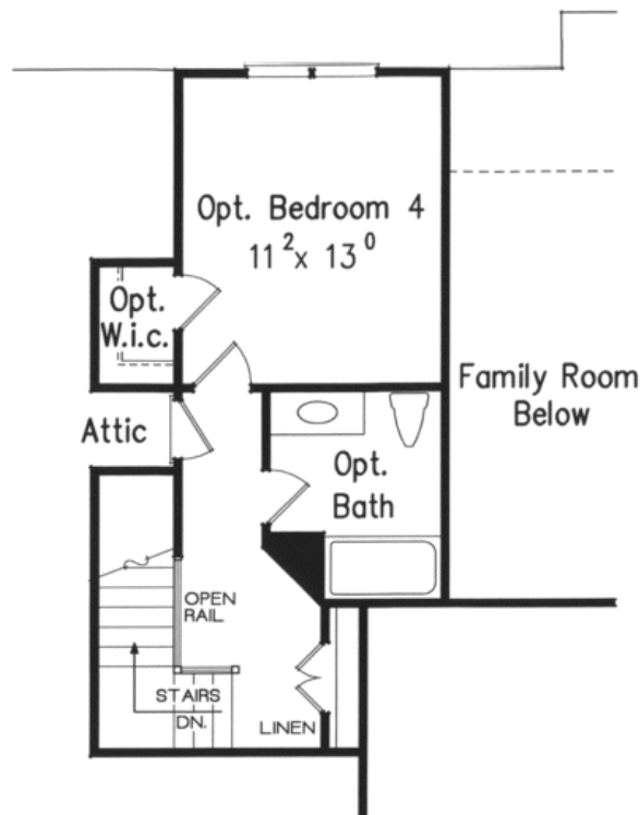
Optional Floor 2
